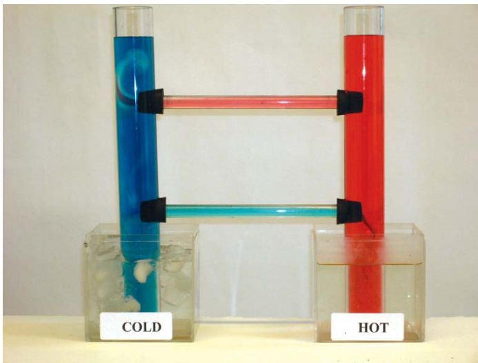
Figure 4.3. Dispositif de convection. Remarquez que l'eau chaude (rouge) circule par le haut tandis que l'eau froide (bleu) circule par le bas dû à la différence de densité entre les deux côtés du dispositif.
