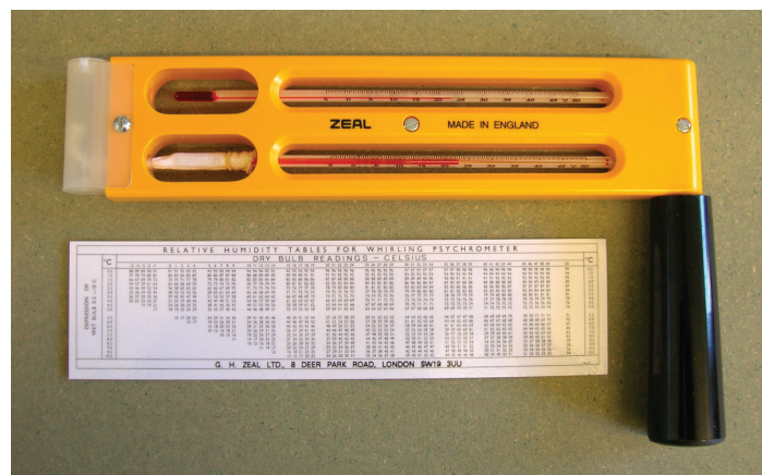
Figura 4.6. Un psicrómetro giratorio y su tabla de conversión.
